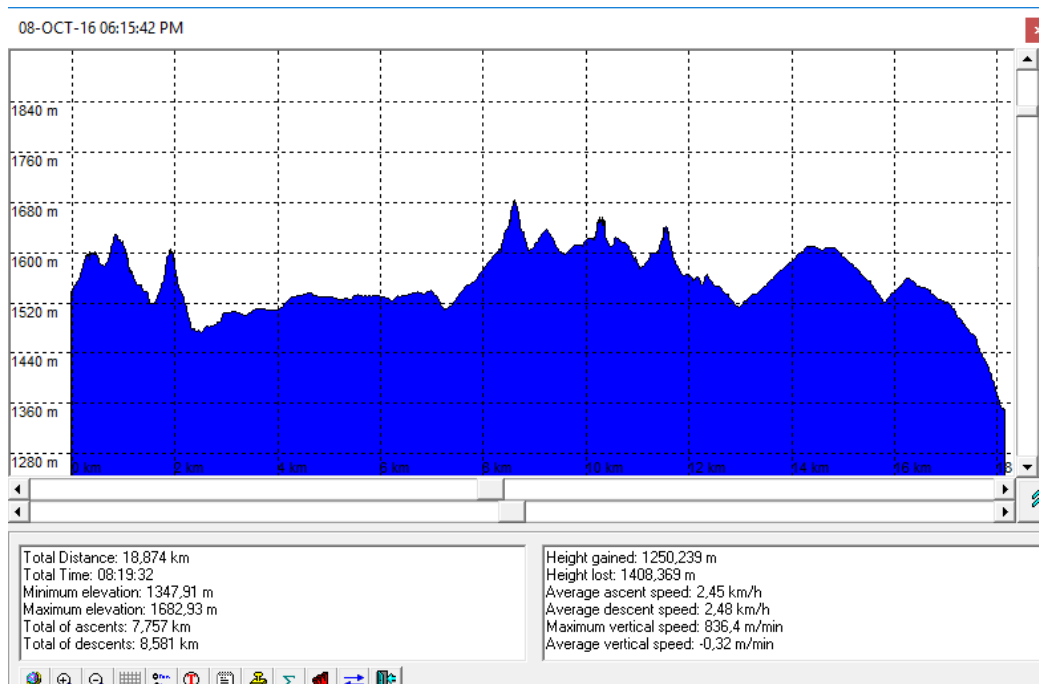
Slika 1 - visinski profil izleta po Premužićevj stazi
